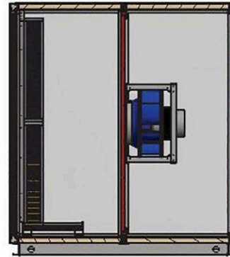
A-A ( 1 : 32 )
